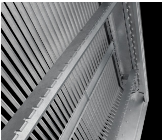
Utbytbara, stavar, spaltvidd och krattelement. Rostfria kedjor och kedjehjul.
